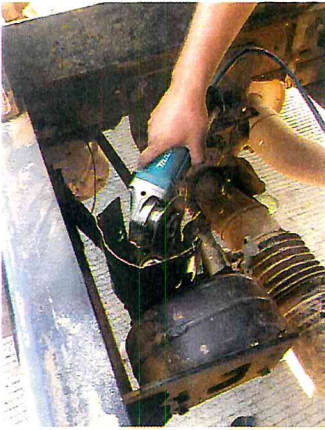
QUITAR VALVULA DE EXCAPE DE AIRE DEL VOLTEO KENWORT
