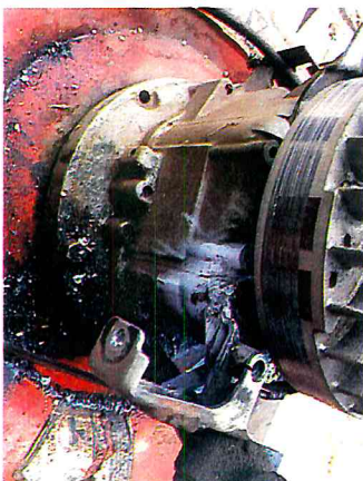
SOLDAR PODADORA DE SERVICIO MUNICIPAL
